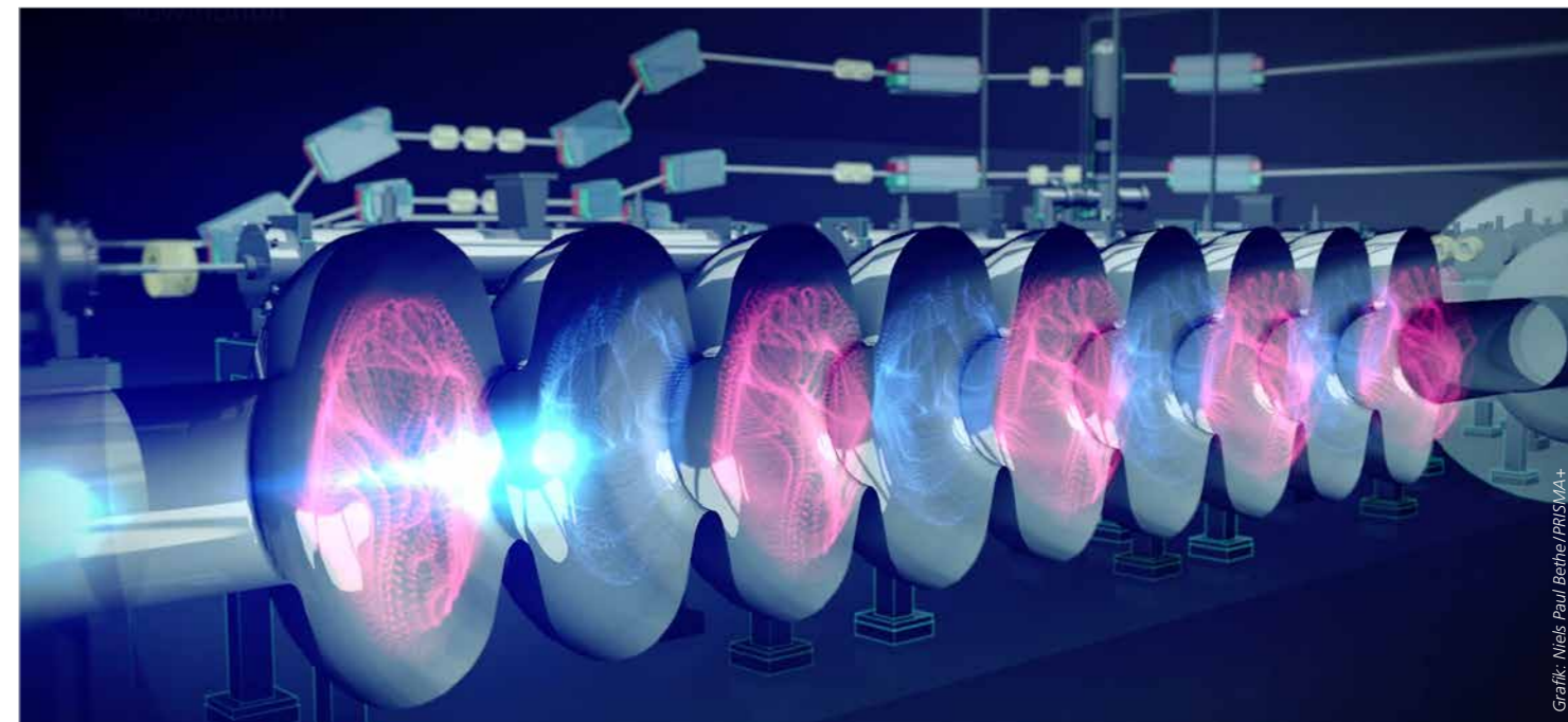
Blick in ein Kryomodul: Im Inneren der „Kavitäten“ werden stehende elektromagnetische Wellen erzeugt. Durch schnelles Umpolen werden diejenigen Elektronen immer weiter beschleunigt, die mit dem Feld synchron fliegen.
